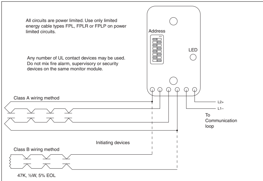
Fig 2. Wiring Diagram for Mini Switch Monitor and Mini Priority Switch Monitor Modules
